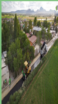
PAVIMENTACIÓN DEL TRAMO LORETO-GUADALUPE DE ATLAS, ASIENTOS
